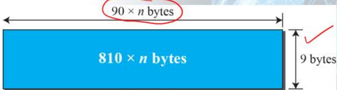
b. STS- n frame
